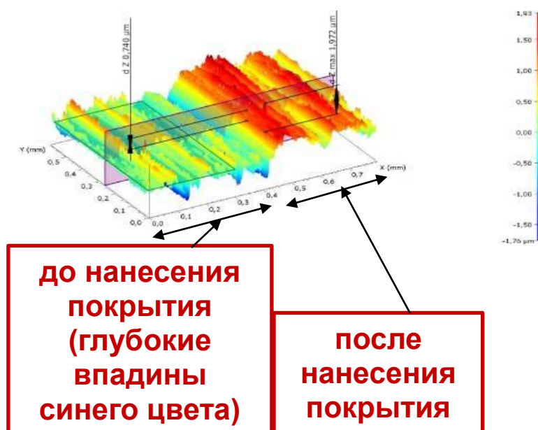
Рис. 7. Трехмерная топография поверхности покрытия BioPateks, где а - до нанесения покрытия видны глубокие впадины синего цвета, б - после нанесения покрытия впадины синего цвета исчезли
