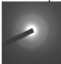
Рис. 2. Электронограмма выделенного участка покрытия BioPateks, характеризующая его аморфность
