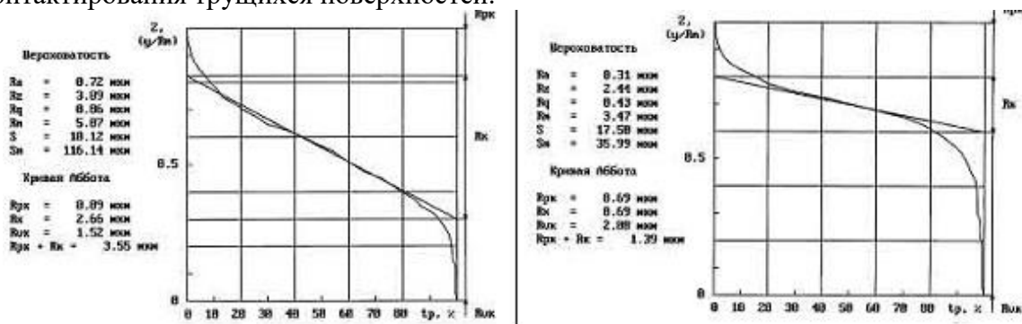
Рис. 5. Кривые опорной поверхности, где а - до нанесения покрытия, б - после нанесения покрытия
