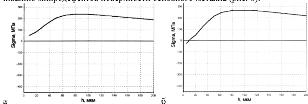
Рис. 6. Эпюры остаточных напряжений поверхности, где а - до нанесения покрытия (шлифованная поверхность с Ra=0,32 мкм), б - после нанесения покрытия
