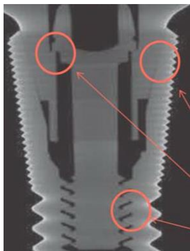
Рис. 1. Зоны фреттинг-коррозии имплантационной конструкции: 1 - зона наружная резьба винта - внутренняя резьба имплантата, 2 - зона упорная полка винта абатмента - упорная поверхность абатмента; 3 - зона наружная конусная поверхность абатмента - внутренняя конусная поверхность имплантата [11]
