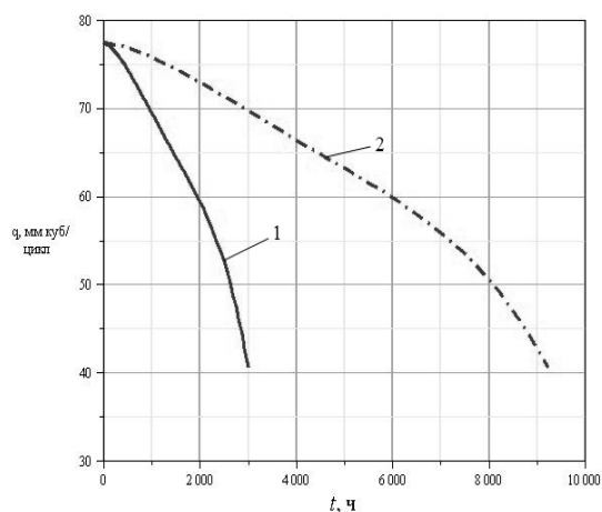
Рисунок 1 – Закономерности характеристик работы ТНВД с заводской плунжерной парой с P_0 = 70 МПа (1) и плунжерной парой с плазменным безвакуумным тонкопленочным покрытием плунжера с P_0 = 160 МПа (2)
